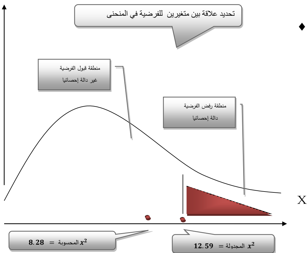
شكل رقم 01 : منحنى يوضح منطقة قبول ورفض مؤشرات الفرضية في مجال تحققها ♣
