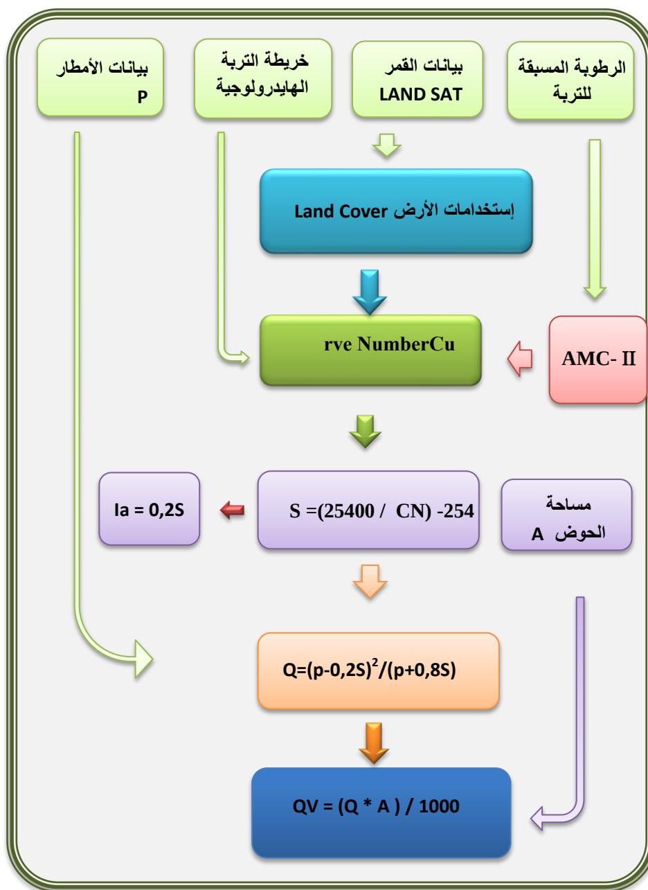
الشكل (1) نموذج عملية تقدير الجريان السطحي وحجم الجريان وفق طريقة ( SCS )
