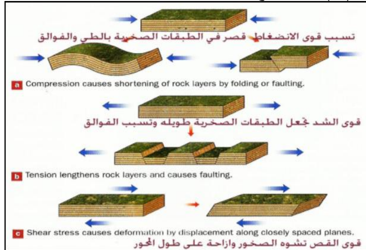
شكل (2) يمثل انواع التشوهات الناتجة عن قوى الاجهاد
