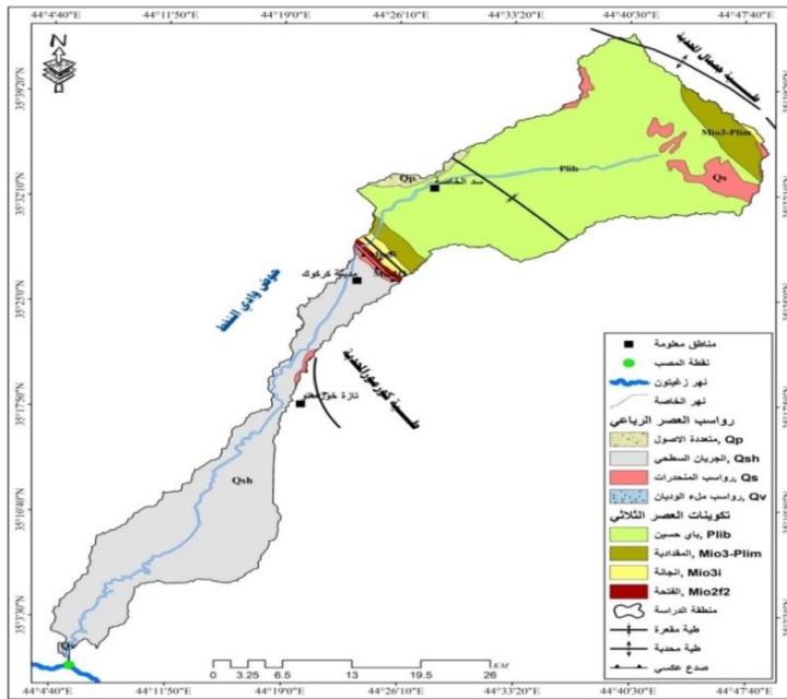
الخريطة (4) جيولوجية منطقة الدراسة
