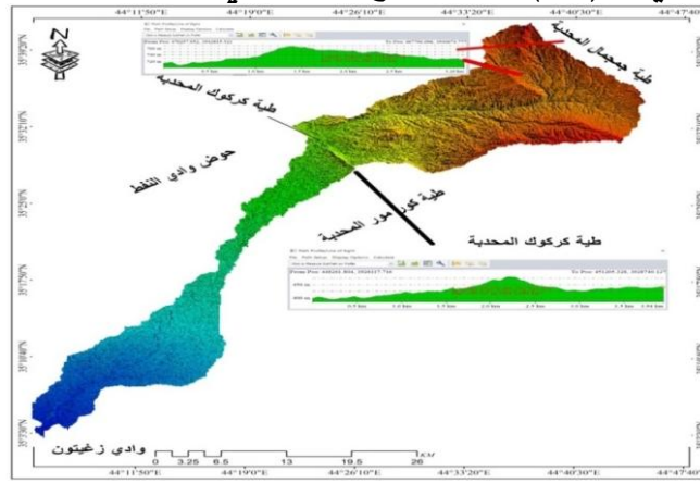
خريطة ( 4 ) شكل وأنواع الطيات في منطقة الدراسة
