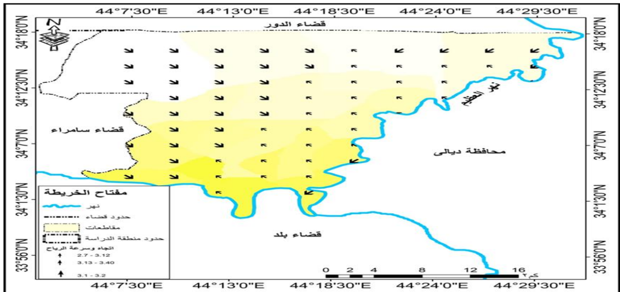
خريطة (3) المعدلات الشهرية والسنوية اتجاه الرياح (م / ثا) لمحطتي سامراء وبغداد لعام 2023
