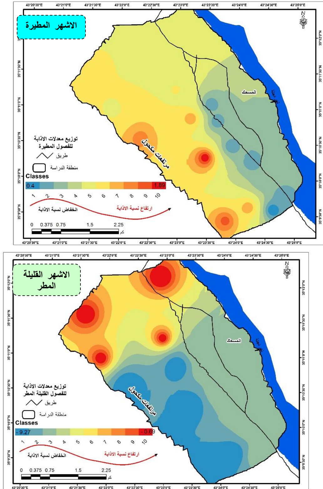
خارطة (7) يوضح معدلات الإذابة لأشهر المطيرة والقليلة المطر لمنطقة الدراسة
