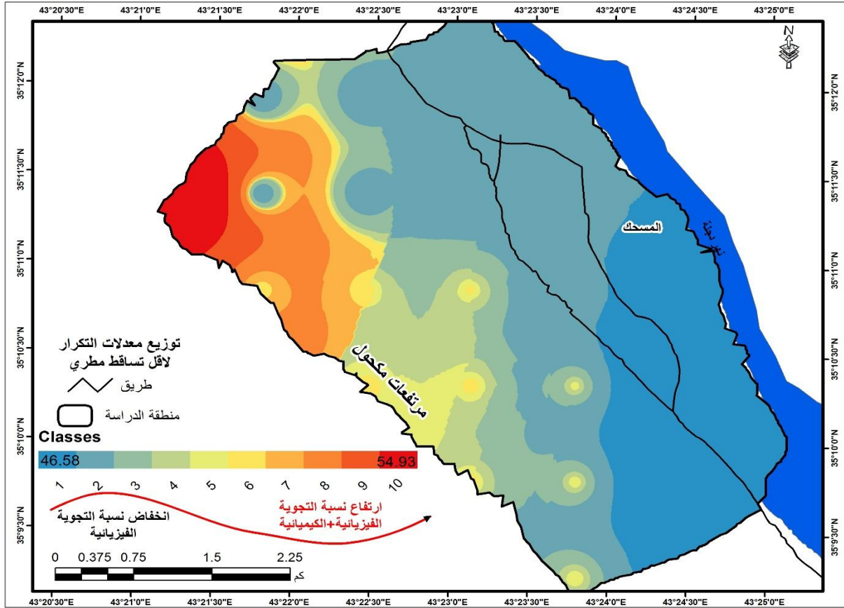
خارطة (4) توضح نسبة تكرار تطرفات تساقط الامطار خلال الاشهر الدافئة لمنطقة الدراسة
