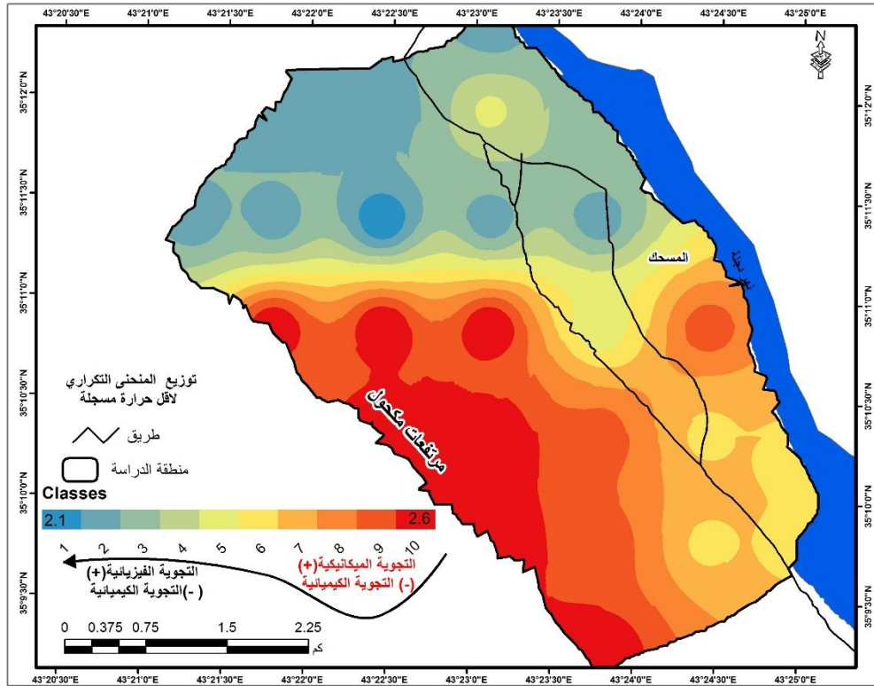
خارطة (6) تمثيل المنحنى التكراري لأقل حرارة مسجلة
