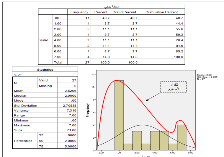
شكل (4) المنحنى التكراري المتوقع لتكون الصقيع لمحطة بيجي
