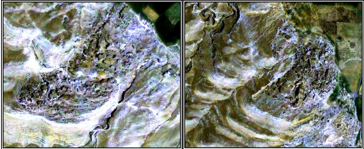
شكل (2) يوضح اثر العواصف المطرية على زحف المواد شمال وشرق المنطقة
