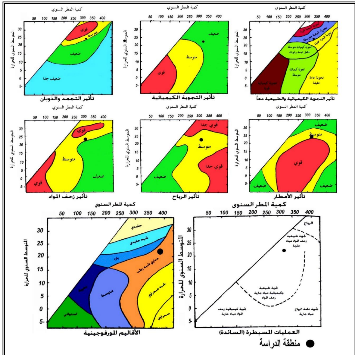
شكل (6) تطبيق نموذج بالتير على منطقة الدراسة
