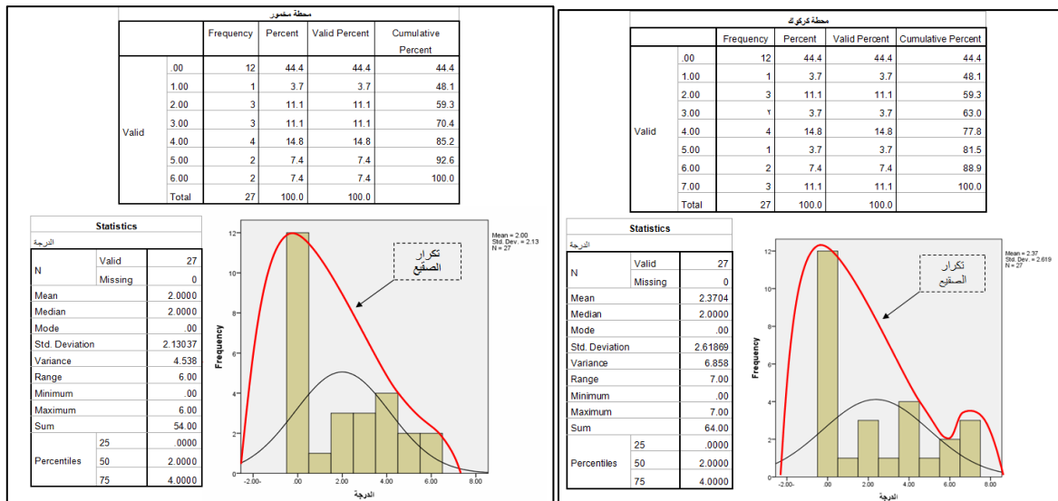
شكل (3) المنحنى التكراري المتوقع لتكون الصقيع لمحطتي مخمور وكركوك
