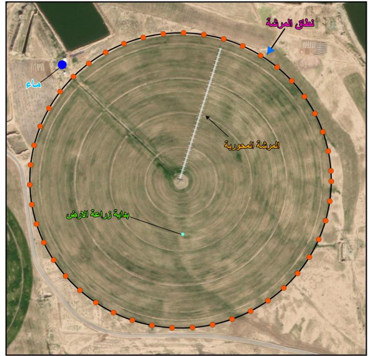
شكل (1): يوضح تصميم ونظام الري المحوري
