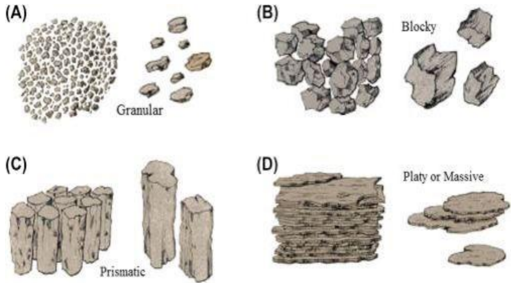
شكل (1) يبين بناء تربة منطقة الدراسة
