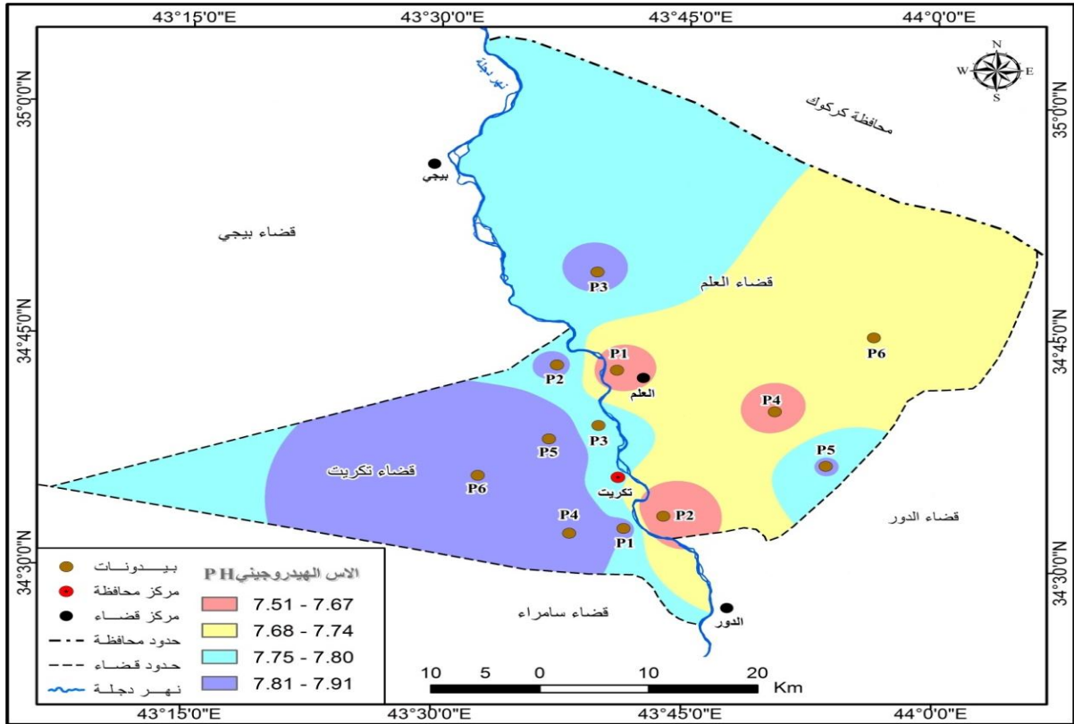
خريطة (4) الأس الهيدروجيني لترب منطقة الدراسة
