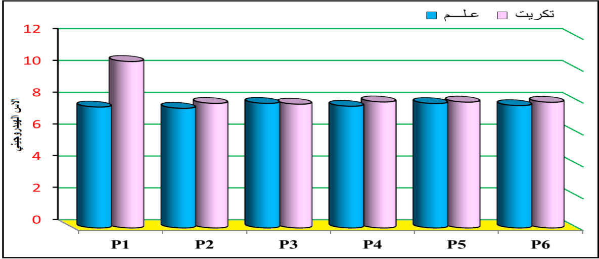
الشكل (4) للأس الهيدروجيني لترب منطقة الدراسة
