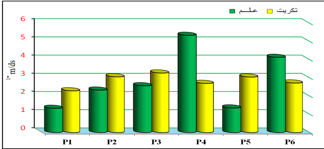
شكل (6) الايصالية الكهربائية لبيدونات منطقة الدراسة
