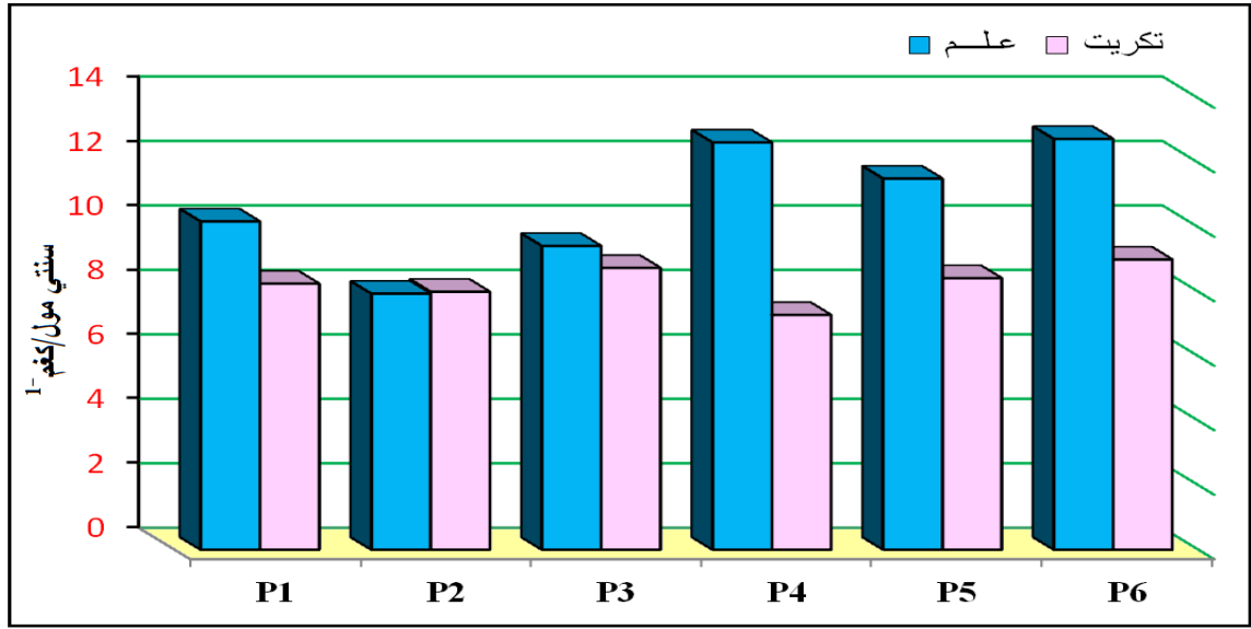
شكل (2) السعة التبادلية الكاتيونية لبيدونات ترب منطقة الدراسة
