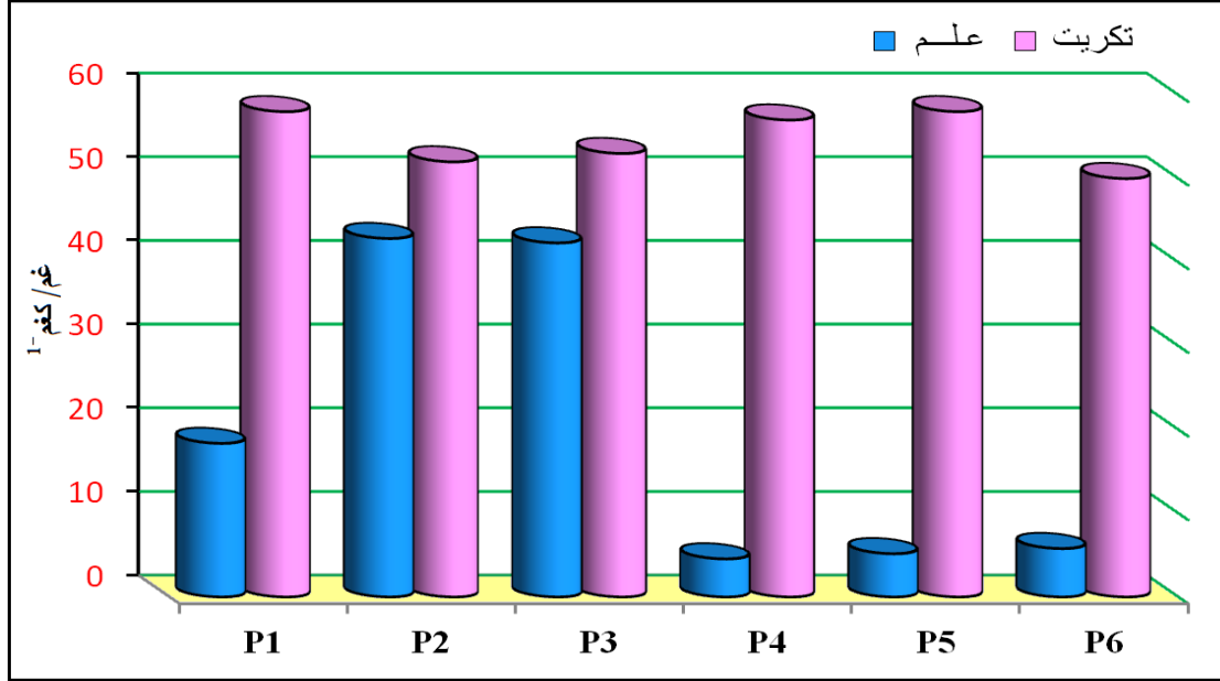
شكل (3) كبريات الكالسيوم لبيدونات منطقة الدراسة
