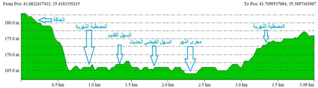
شكل (5) حافات المصاطب النهرية في منطقة الدراسة للموقع (B)
