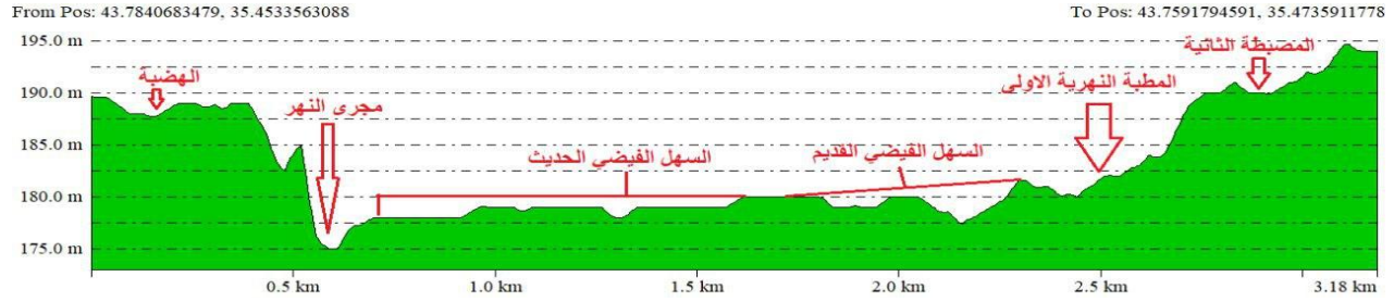
شكل (4) المصبطة النهرية الاولى والثانية لنهر الزاب الاسفل في منطقة الدراسة للموقع (A)
