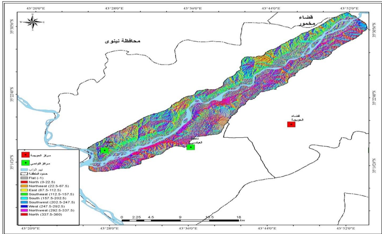
خريطة (5) اتجاه الانحدار السطح منطقة الدراسة
