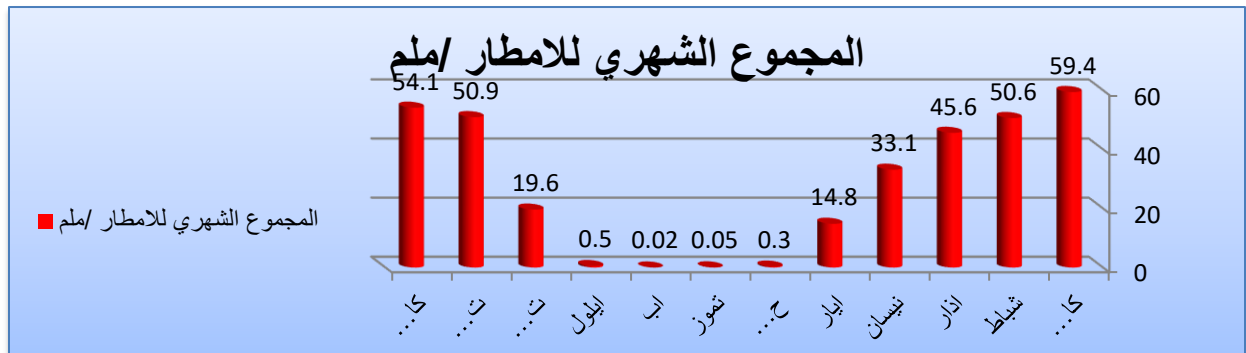
شكل (3) مجموع كمية المعدلات الشهرية لكمية الامطار (ملم) في محطة كركوك للمدة (1990-2022م)
