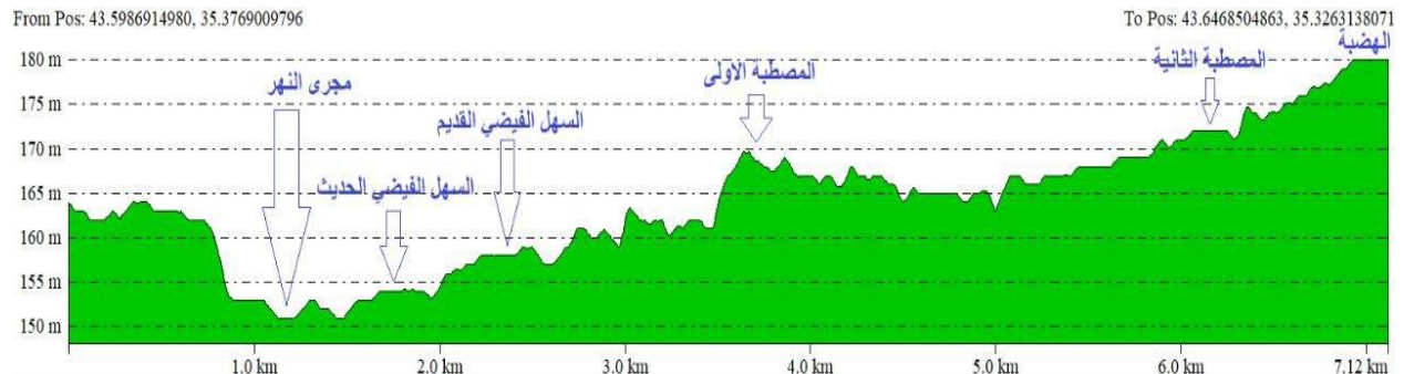
شكل (6) المجرى النهر لنهر الزاب الأسفل في منطقة الدراسة للموقع (C)
