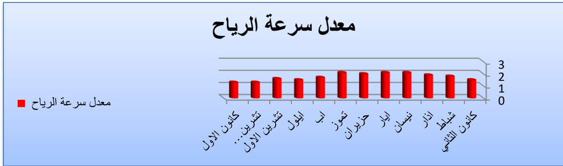
شكل (2) معدل سرعة الرياح في محطة كركوك (م/ثا) للمدة (1990.2022م)
