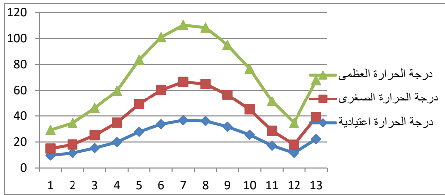
شكل (1) متوسطات درجات الحرارة (درجة مئوية) في محطة كركوك للمدة (1990-2022)
