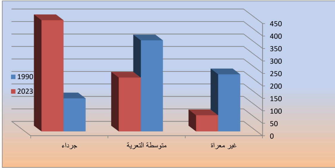
شكل(3) مساحة مؤشر دليل التربة العارية (BSI) لمنطقة الدراسة للمدة (1990-2023)
