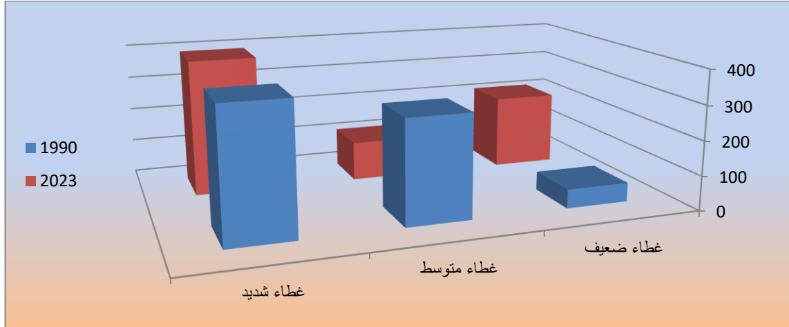
شكل (1) مساحة مؤشر دليل الاختلاف النبات الطبيعي الاخضر (GNDVI) لمنطقة الدراسة للمدة (1990-2023)
