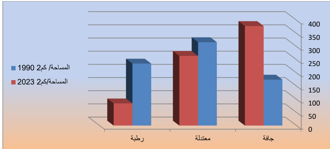
شكل (4) نسب مؤشر دليل الاختلاف الطبيعي للرطوبة (NDMI) لمنطقة الدراسة للمدة (2023-1990)
