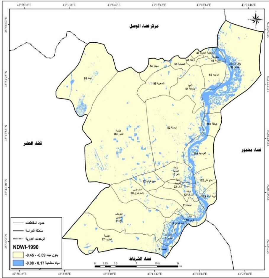
المصدر: من عمل الباحثة اعتماداً على المرئية الفضائية ( Landsat 5 Mss ) ومخرجات برنامج (Arc Map 10.7) بتاريخ 1990/3/24.
