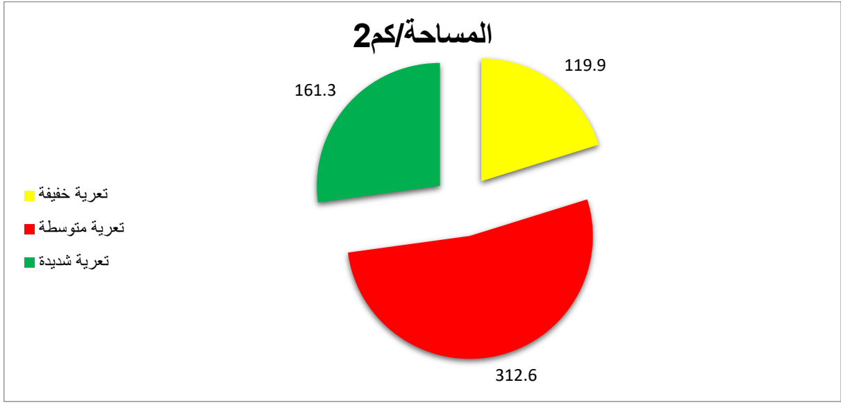
شكل (3) انواع التعرية ومساحتها (م/كم 2 )
