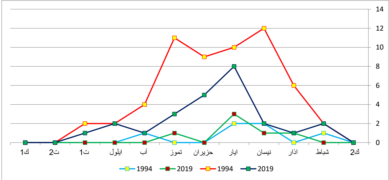
شكل (1) تكرار ظواهر الجو الغبارية (يوم) في منطقة الدراسة لمحطة مخمور لعامي 1994 - 2019
