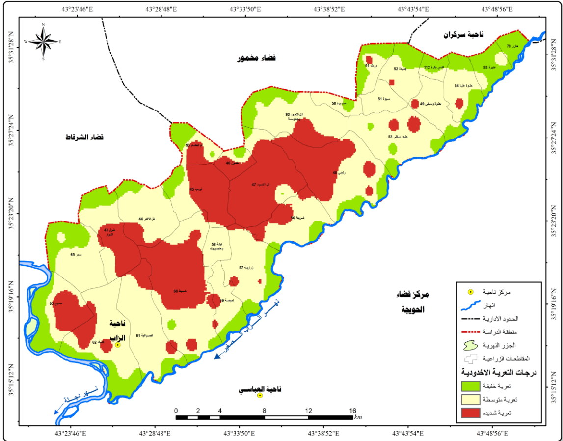
خريطة (2) تصنيف درجات التعرية الأخرودية في منطقة الدراسة
