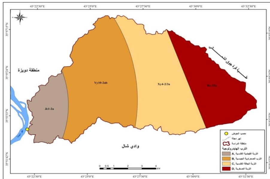
خريطة (3) هيدرولوجية التربة في منطقة الدراسة
