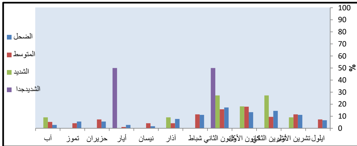
شكل (10) النسب المئوية لعدد ايام بقاء شدة الانقلاب الحراري السطحي فوق مدينة الدمام الصناعية للمدة 2011-2022
