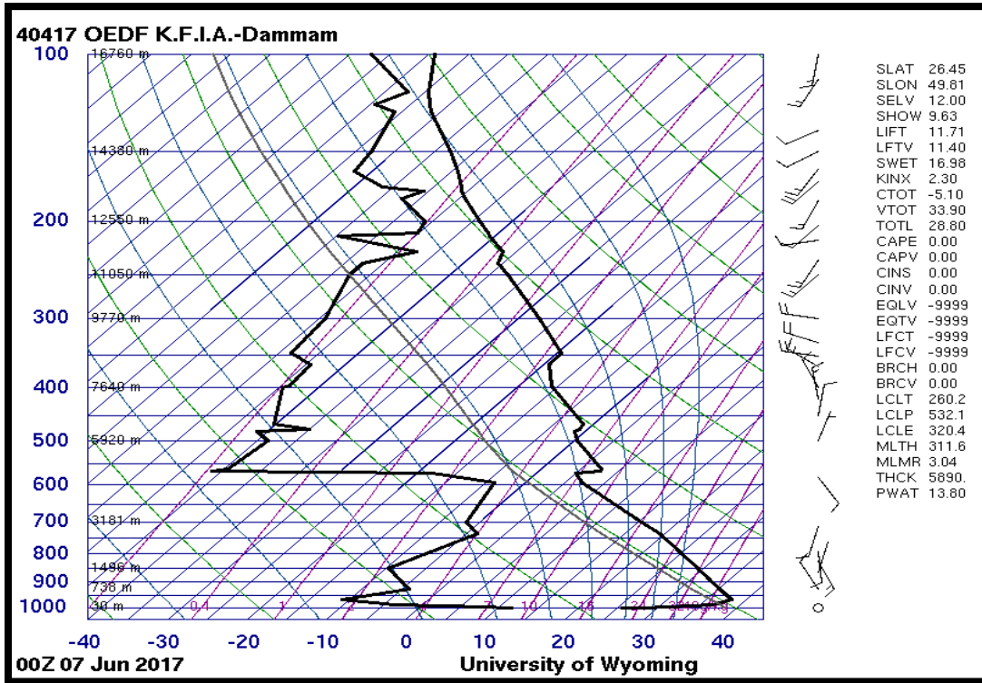
شكل (3) مخطط دايجرام ليوم 2017/6/7 الرصدة 00 توضح انقلابا حراريا سطحيا فوق مدينة الدمام
