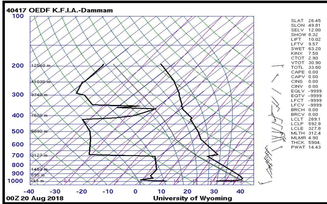
شكل ( 6 ) مخطط دايجرام ليوم 2018/8/20 الرصدة 00 توضح انقلابا حراريا علويا فوق من النوع الهبوطي فوق مدينة الدمام
