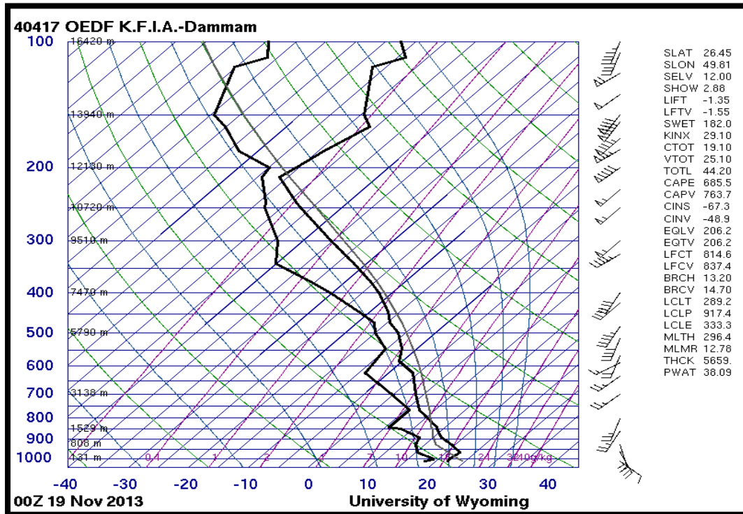
شكل ( 7 ) مخطط دايجرام ليوم 2013/11/91 الرصدة 00 توضح انقلابا حراريا جبهيا فوق من النوع الجبهي فوق مدينة الدمام
