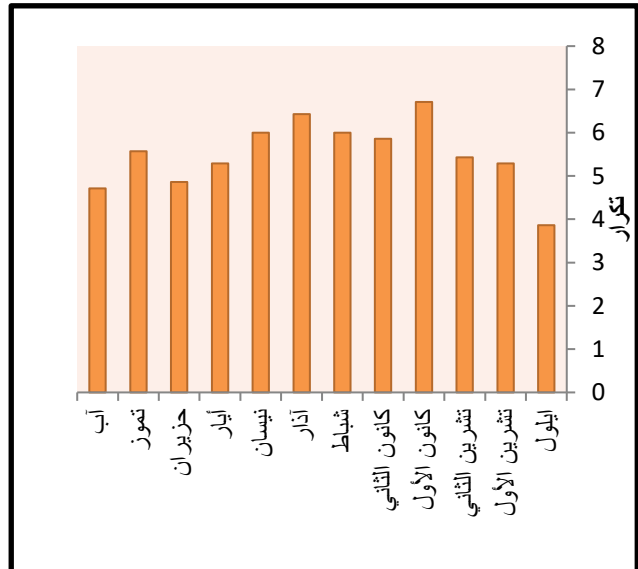
شكل (1) المعدلات الشهرية لتكرار الانقلاب السطحي فوق مدينة الدمام للمدة 2011-2021
