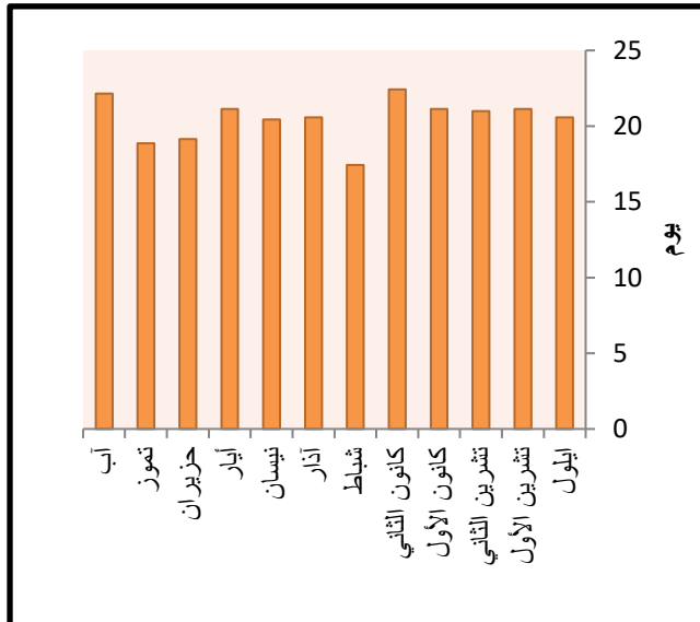
شكل (2) المعدلات الشهرية لعدد ايام الانقلاب فوق مدينة الدمام للمدة 2011-2021
