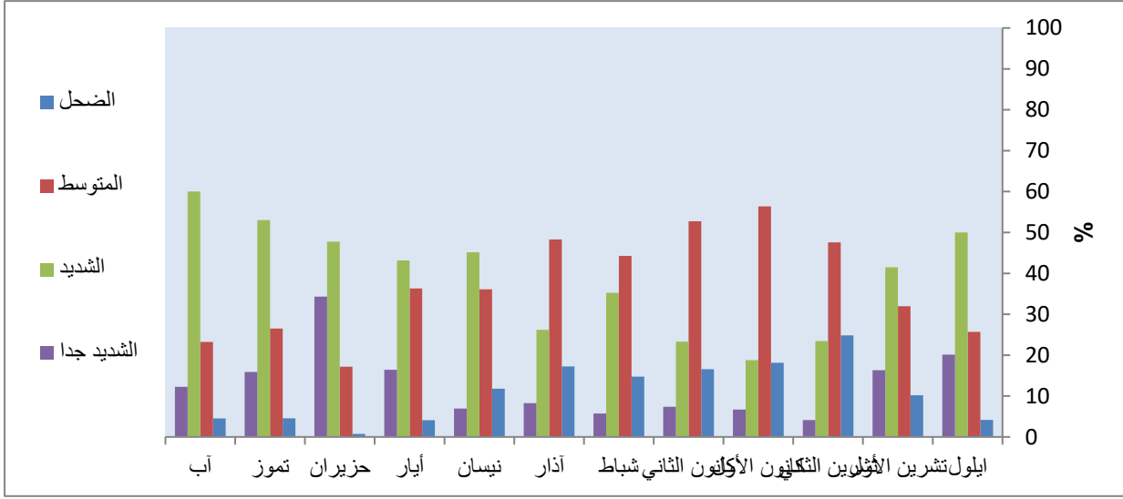
شكل (11) النسب المئوية لعدد ايام بقاء الانقلاب الحراري العلوي فوق مدينة الدمام الصناعية للمدة 2011-2022
