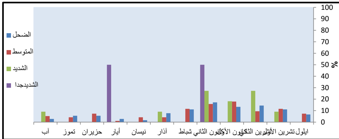
شكل (10) النسب المنوية لعدد ايام بقاء شدة الانقلاب الحراري السطحي فوق مدينة الدمام الصناعية للمدة 2011-2022
