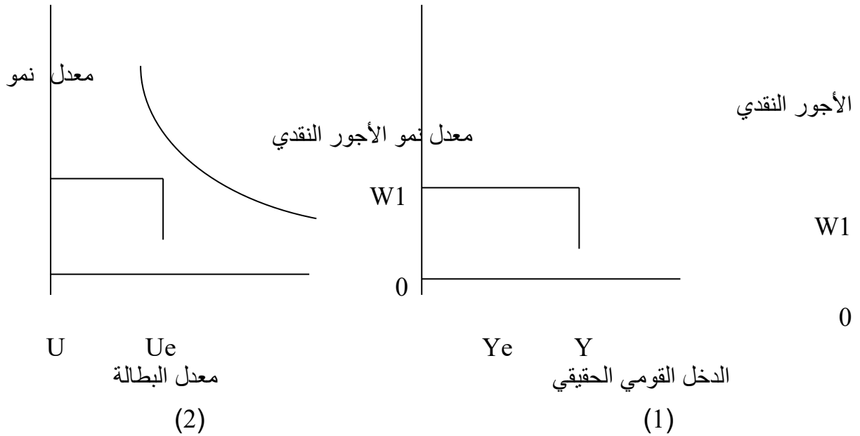
الشكل الثاني: علاقة منحى فيليبس بالدخل القومي (26)
