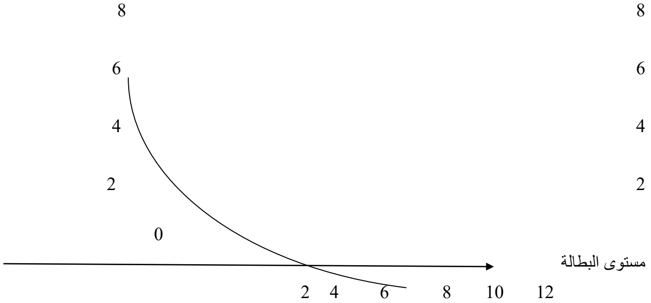
الشكل الثاني: علاقة منحى فيليبس بالدخل القومي (26)
