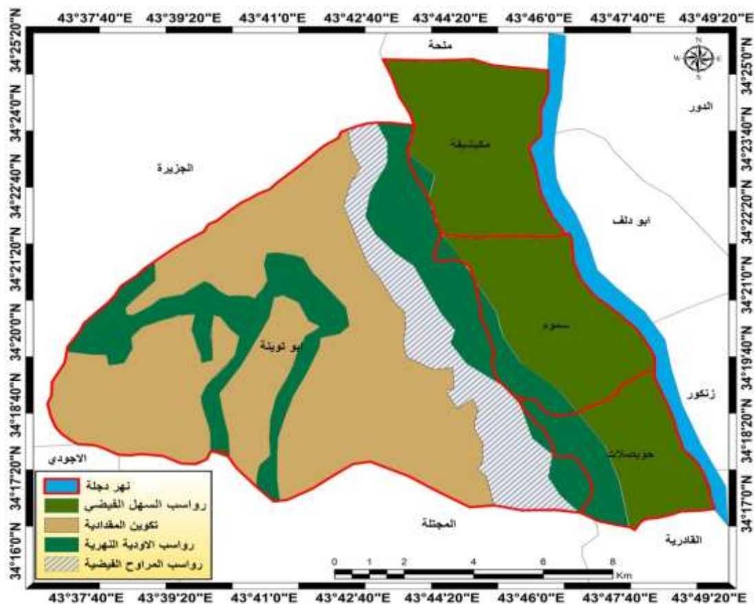
خريطة (2) الاقسام الجيولوجية لمنطقة الدراسة
