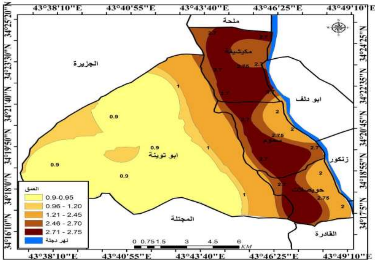
خريطة ( 3 ) عمق التربة
