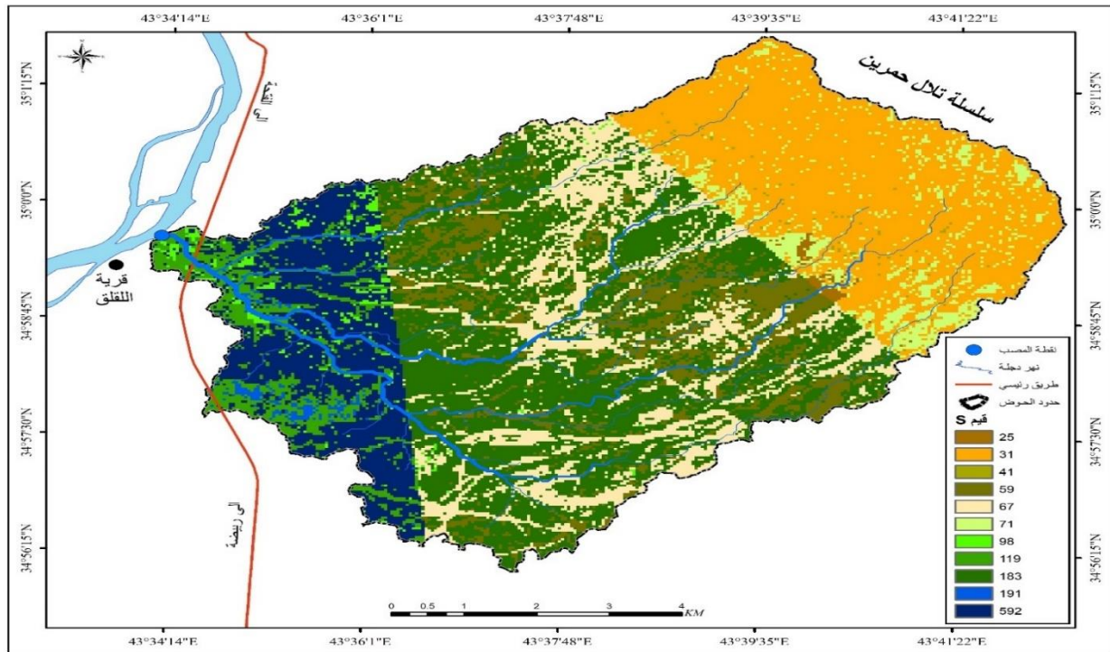
خريطة (5) تبين قيم (S) لحوض منطقة الدراسة
